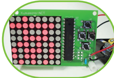
LED電光掲示板製作
